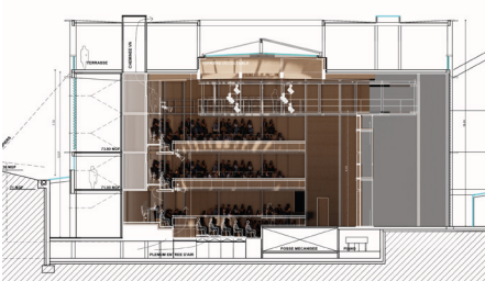
Coupe du théâtre • 2024 • ©Studio Andrew Todd
